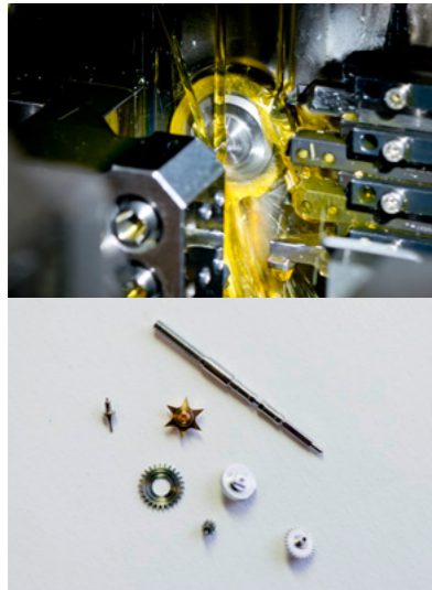
Décolletage des pignons et planches de roues Pinions and wheels cutting
